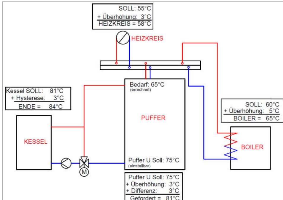
Obr. 8.3. Teplotný manažér s akumuláčnym zásobníkom a s diferenciou
