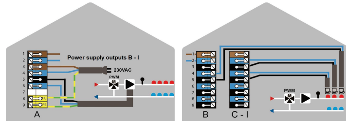
Sieťové pripojenie obehového čerpadla vyk. okruhu.
