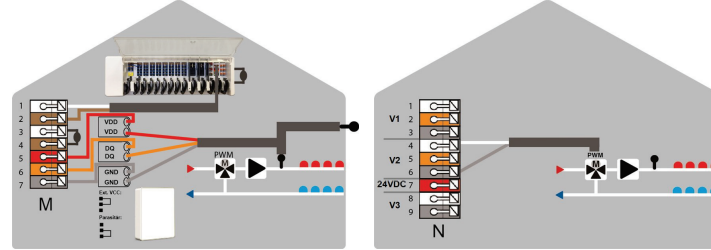
CAN-Bus budovy a 1-vodičové snímače
