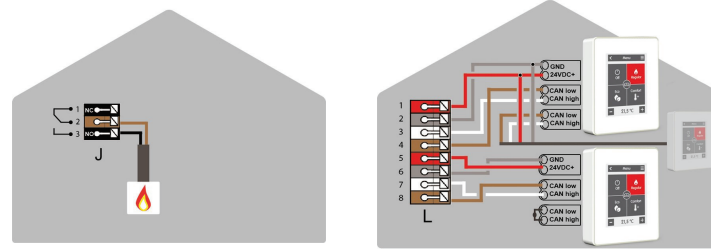
Bezpotenciálové prepínacie kontakty pre ďalšie funkcie
